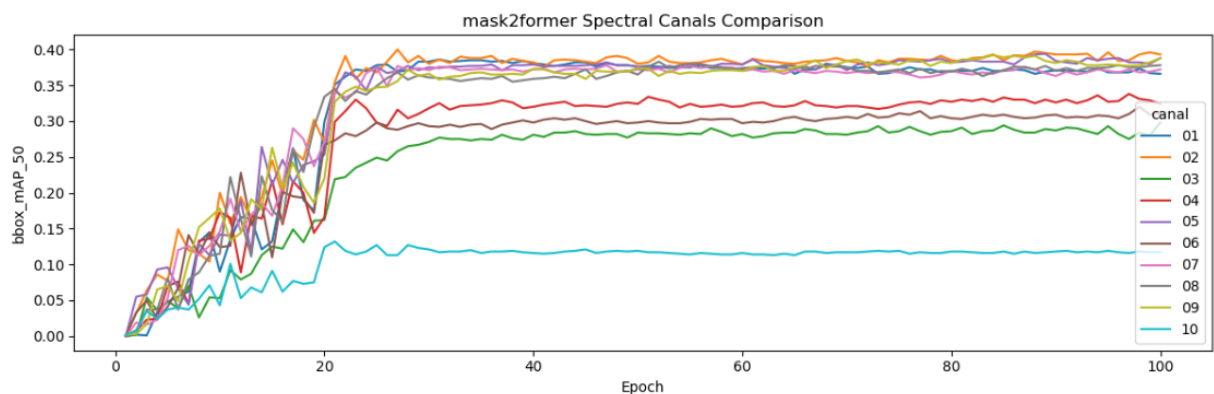
Rysunek 4.12. Porównanie wyników modelu Mask2Former trenowanego na poszczególnych kanałach spektralnych.
