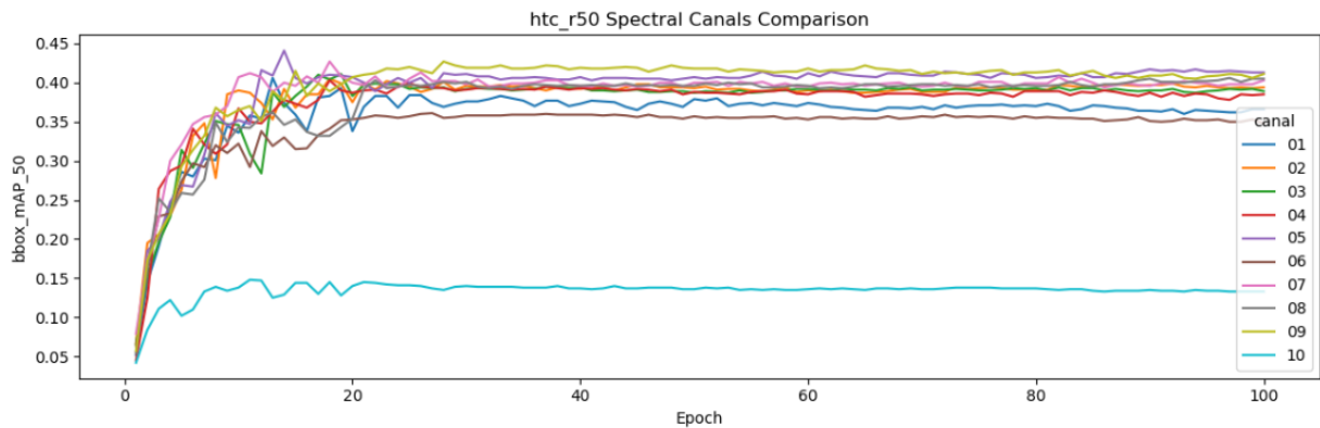
Rysunek 4.11. Porównanie wyników modelu HTC_r50 trenowanego na poszczególnych kanałach spektralnych.
