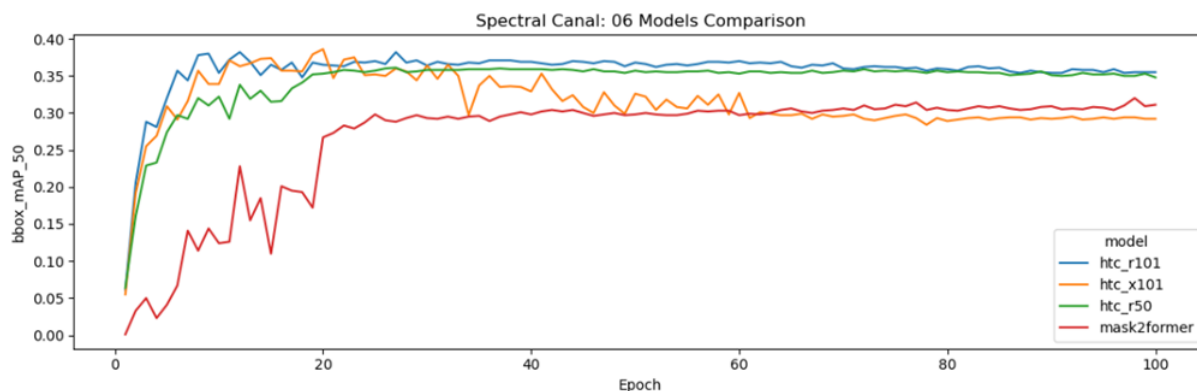
Rysunek 4.20. Porównanie przebiegu trenowania poszczególnych modeli na zbiorze danych z szóstego kanału spektralnego.
