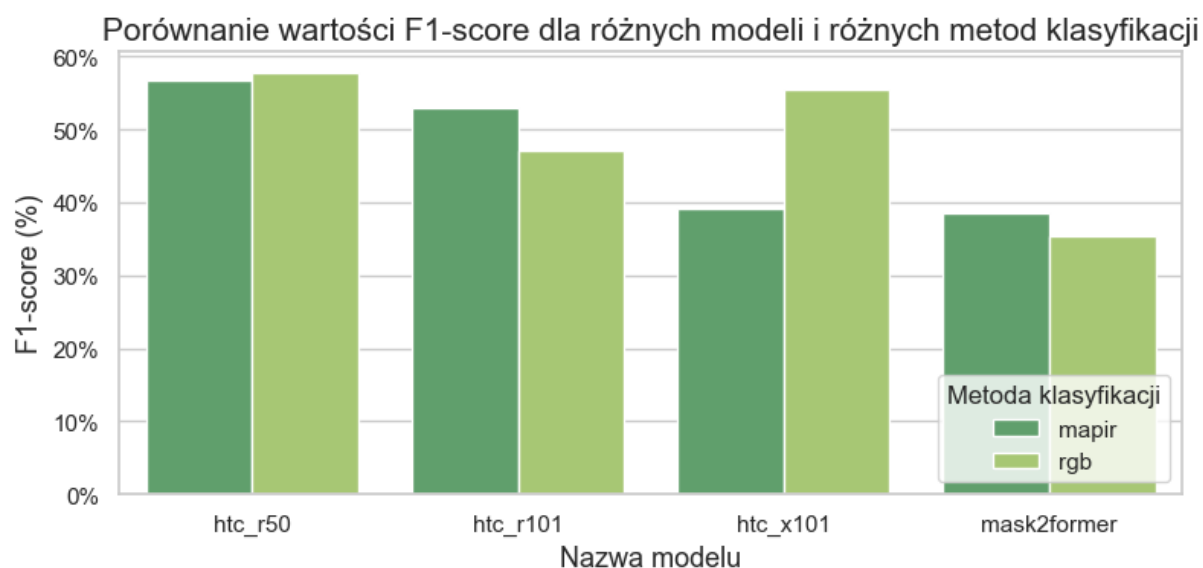
Rysunek 5.2. Wykres przedstawiający wartości parametru F1-score dla poszczególnych algorytmów oraz analizowanych typów zobrażenia: RGB oraz wielospektralnego z kamery MapIR Survey3 Red+Green+NIR.
